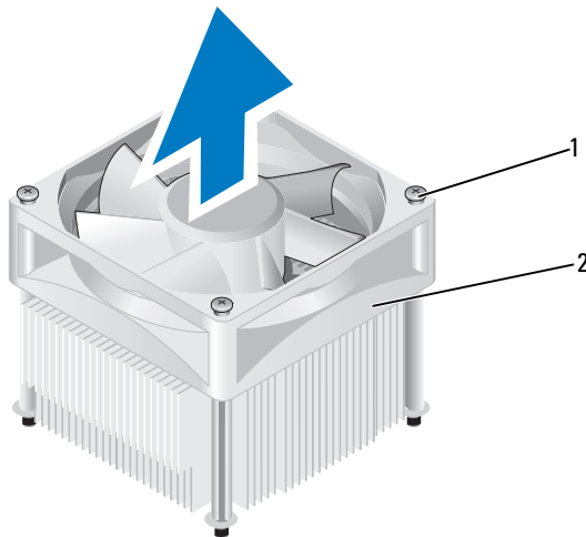
1 fästskruvar (4) 2 processorfläkt/kylfläns
